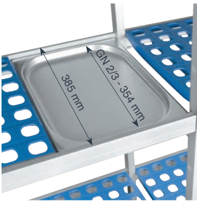
Fondo · Width: 385 mm Altura · Height: 2.000 mm
